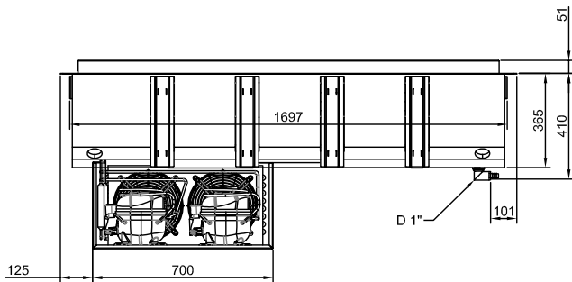
Achterzijde
